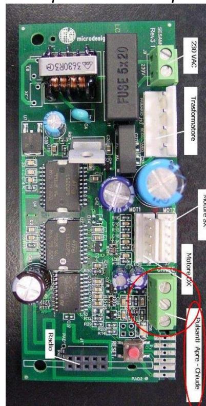
Morsetti per i tre cavi dei pulsanti
